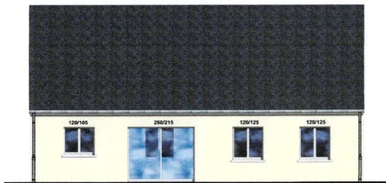
FACADE NORD
